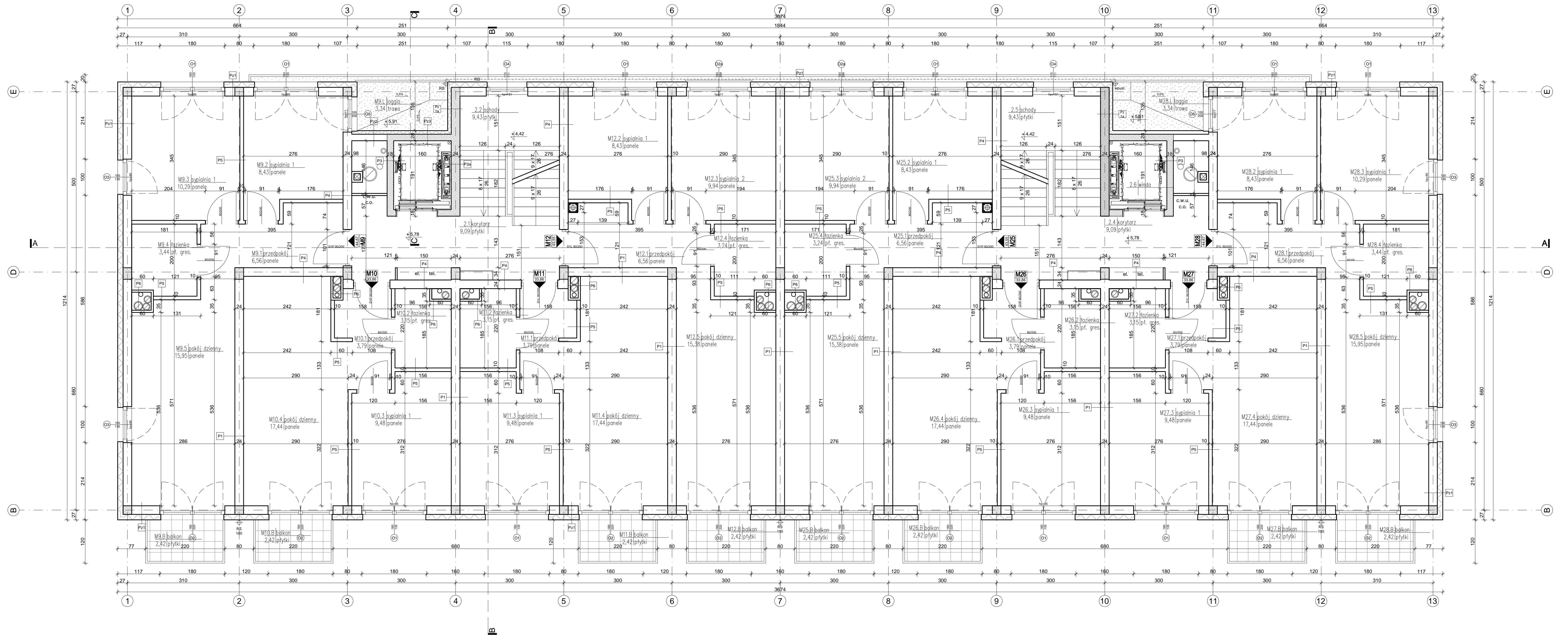
BUDYNEK E - RZUT 2 PIĘTRA
