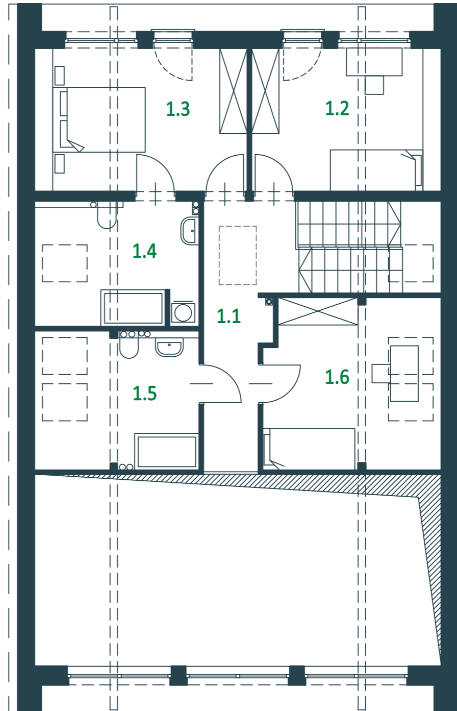
RZUT PODDASZA
