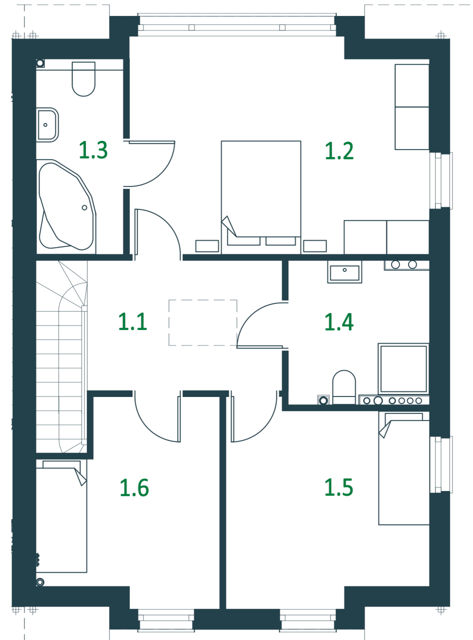
RZUT PODDASZA
