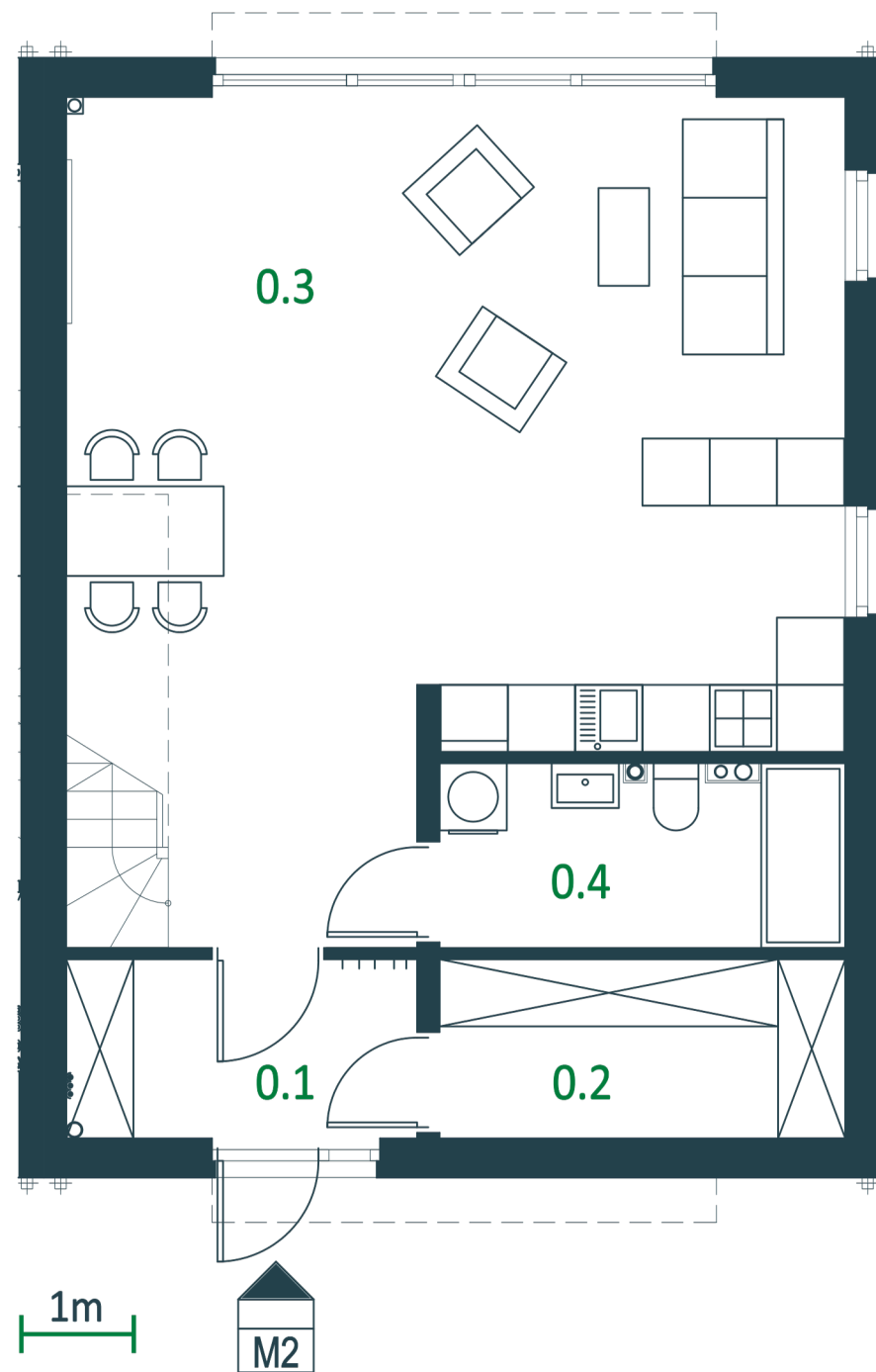
RZUT PARTERU
